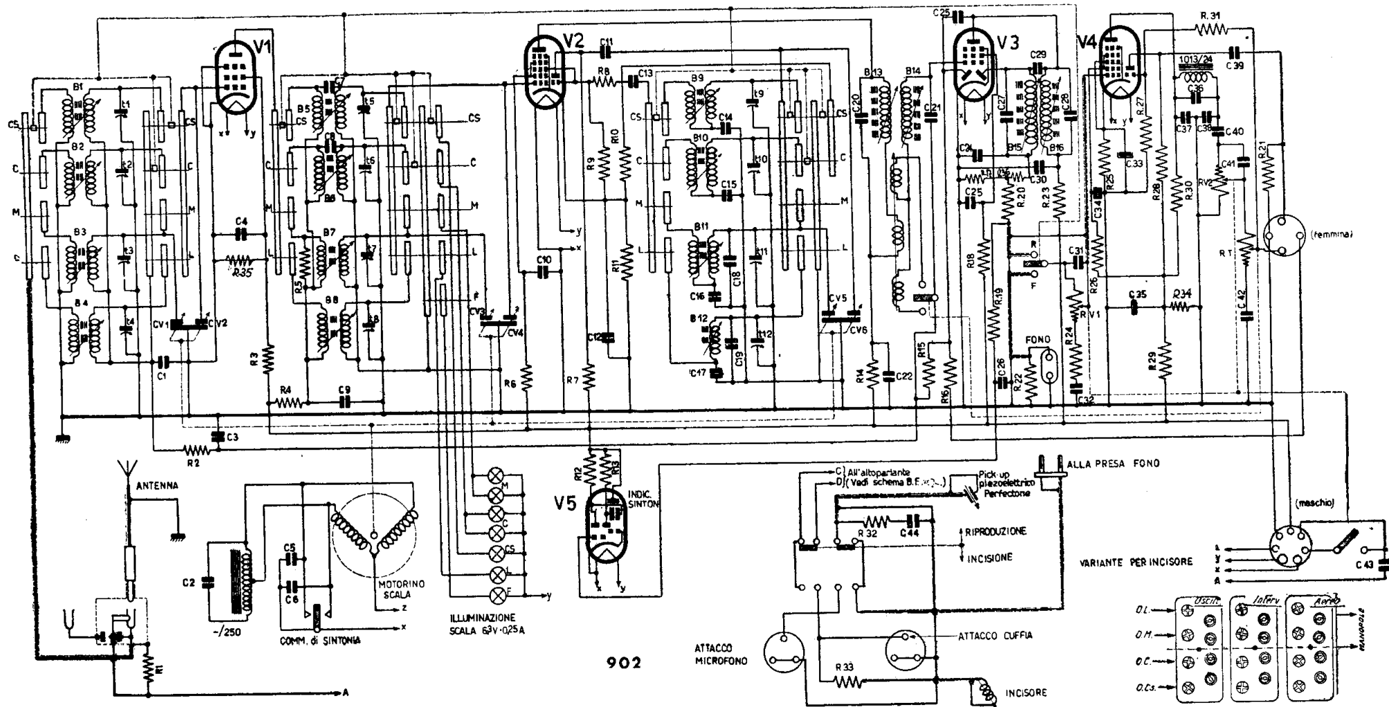
PHONOLA RADIO - Mod. 902 - Lunghe da 2000 a 927 m, medie da 600 a 187 m, corte da 51,7 a 23 m, cortissime da 23,4 a 11,4 m. Media frequenza 470 kc/s. Posizione compensatori v. schema mod. 625. Potenza d'uscita 10 W. Consumo 120 W. (Per valvole v. schema BF, per tensioni v. tabella mod. 625).
